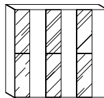
FASCIA 3 Ante L.273 X P.66 X H.258
